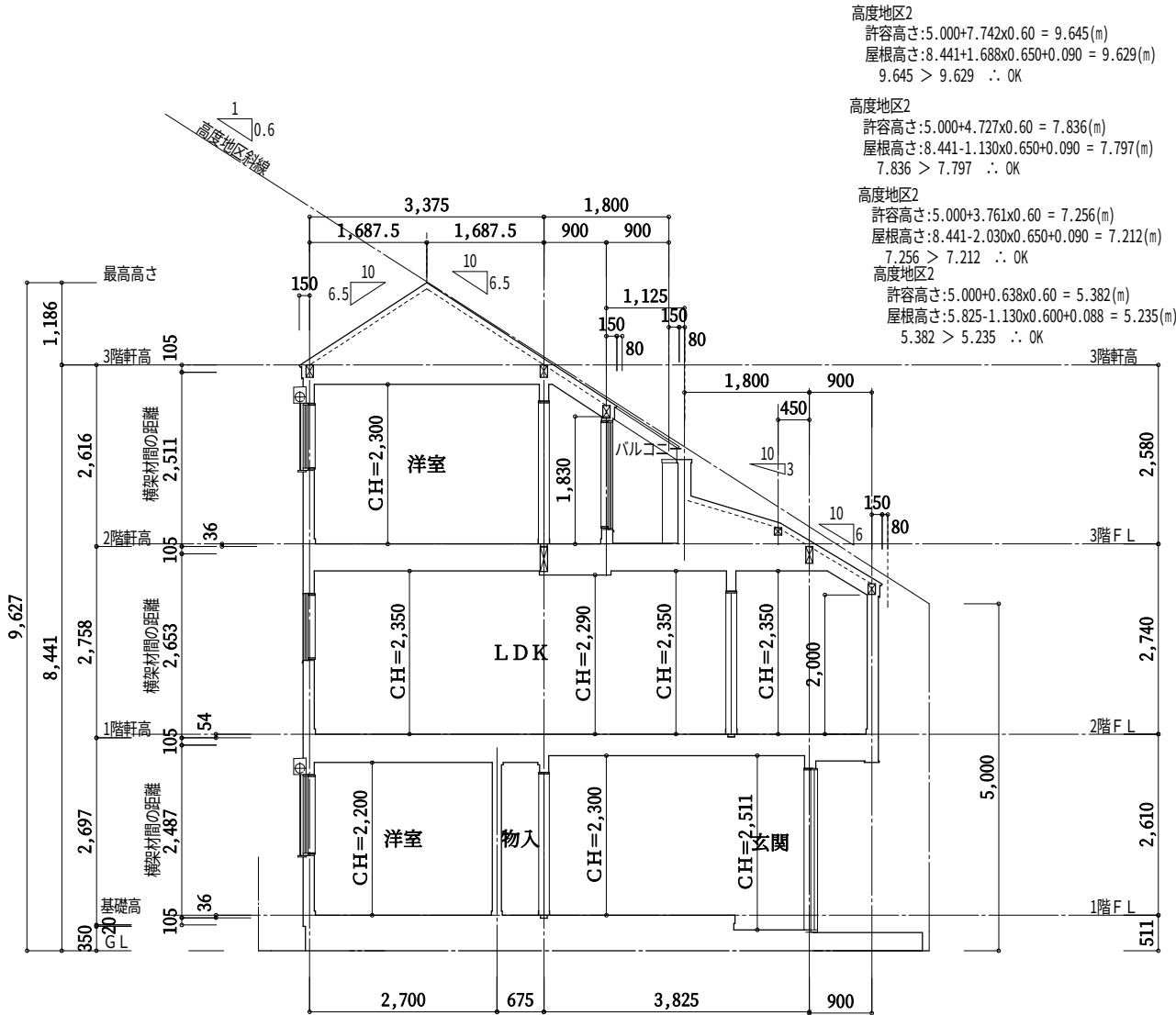
1面 断面図
