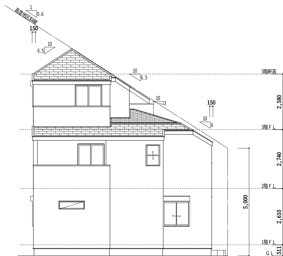
東側 立面図
