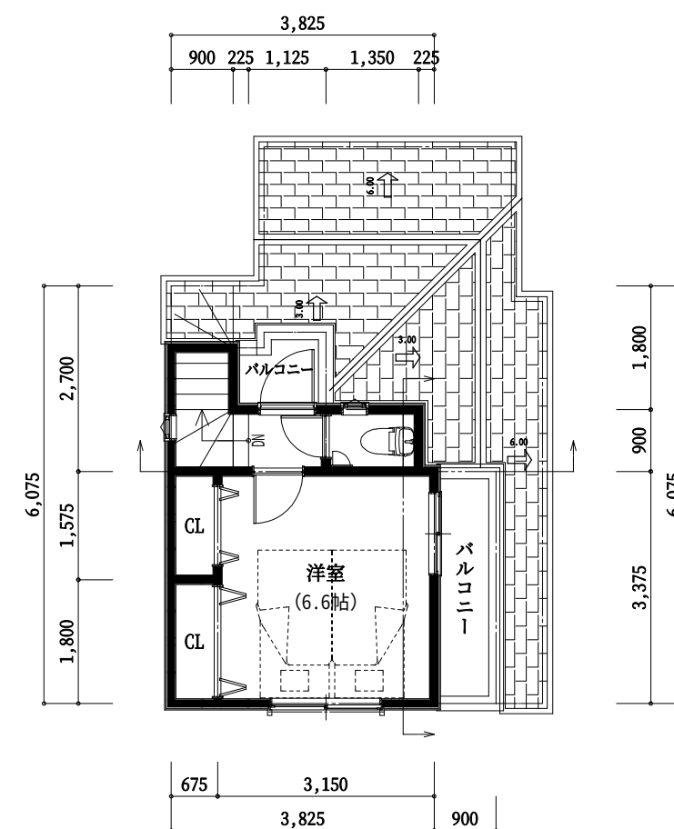
3階 平面図
