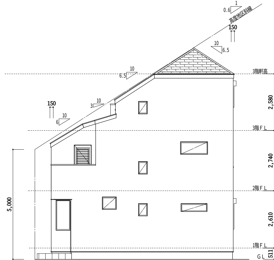
西側 立面図
