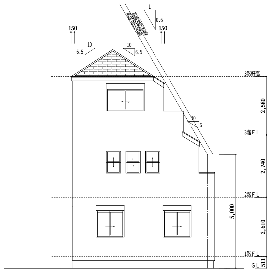
南側 立面図
