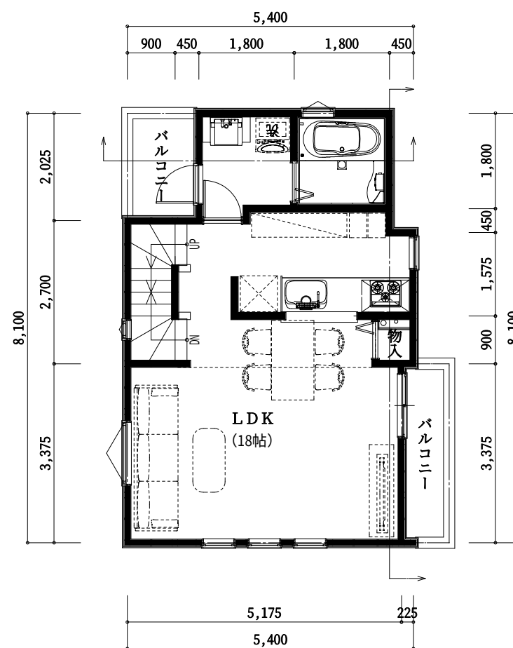
2階 平面図
