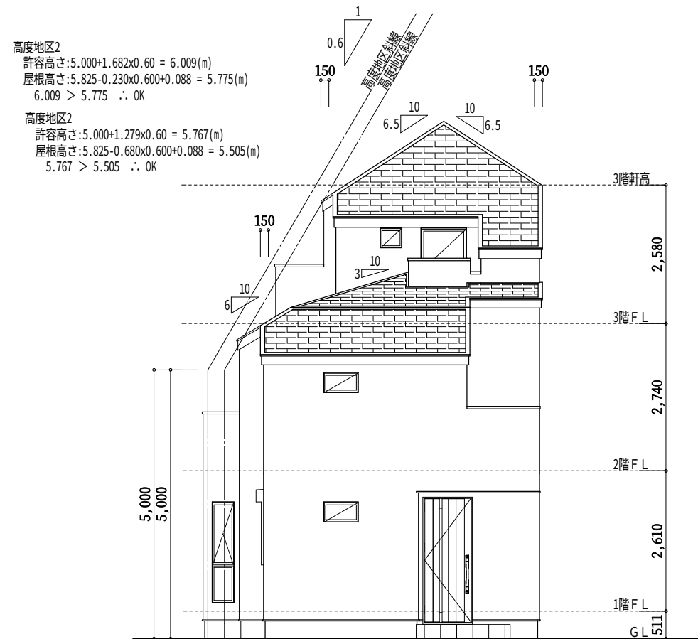
北側 立面図
