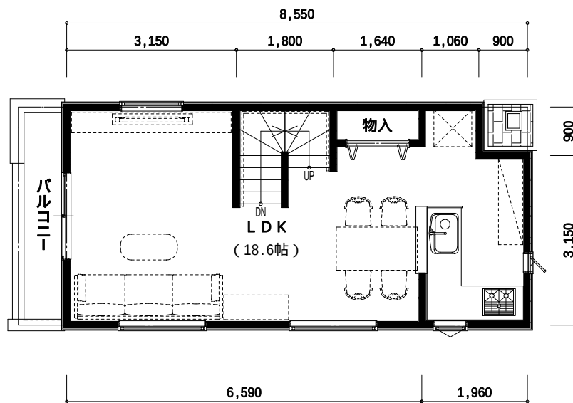
2階 平面図
