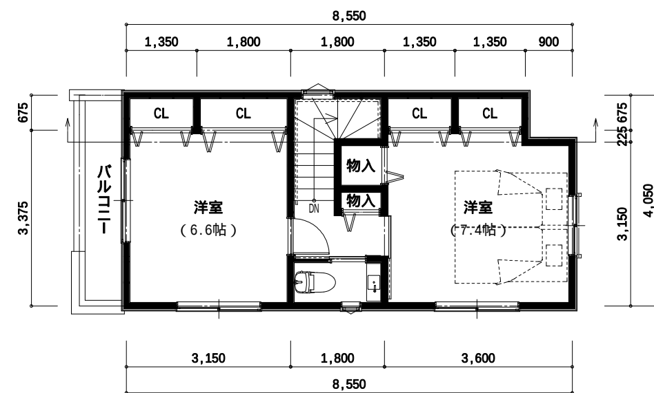
3階 平面図
