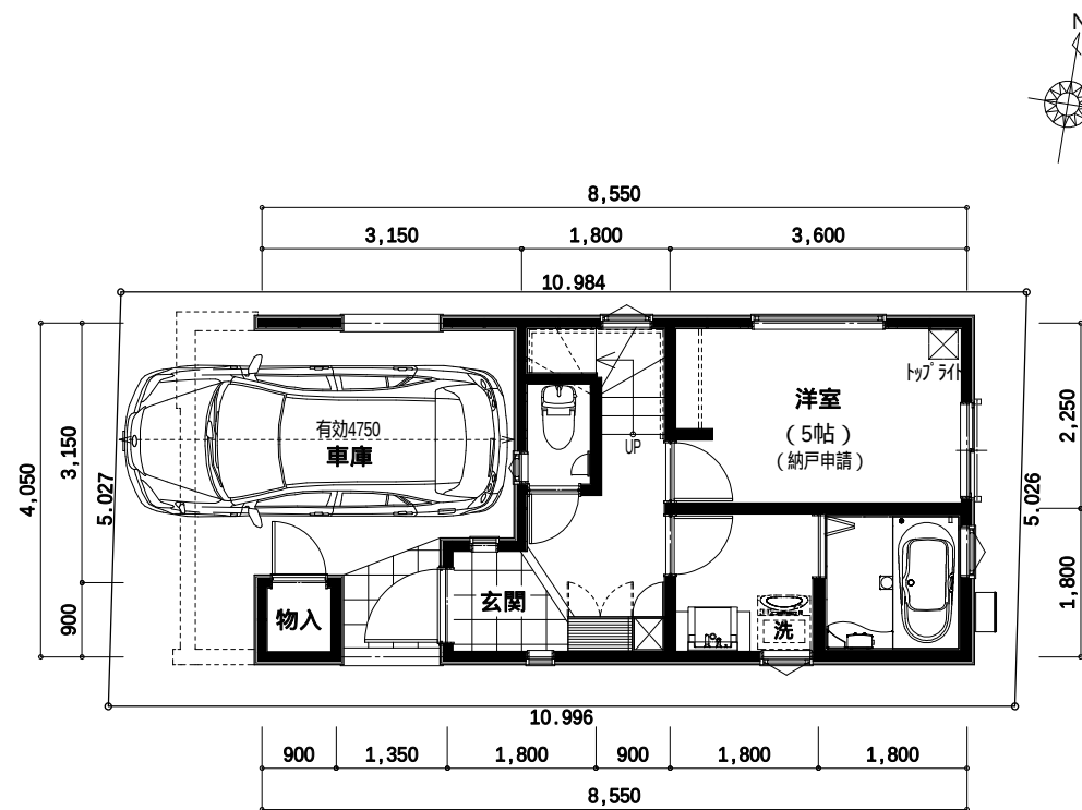
1階 平面図
