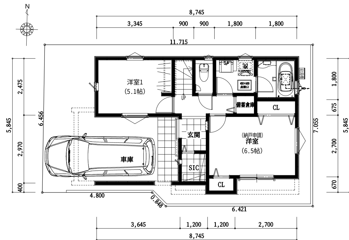
1階 平面図
