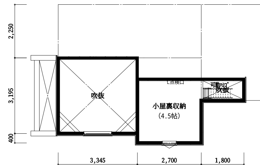
R階 平面図
