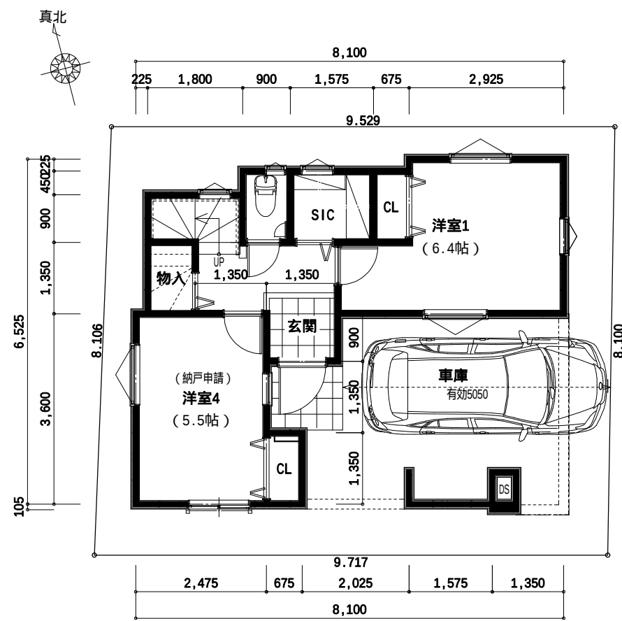
1階 平面図
