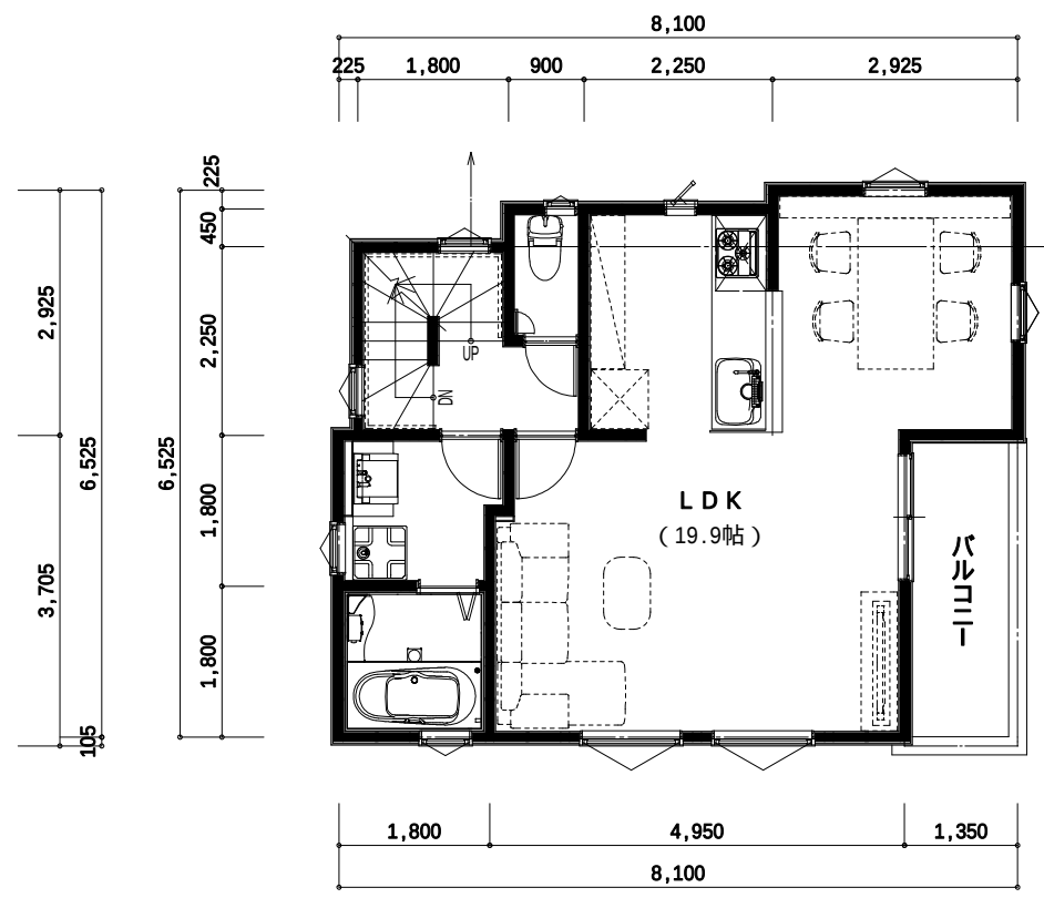
2階 平面図
