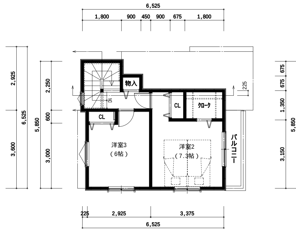
3階 平面図
