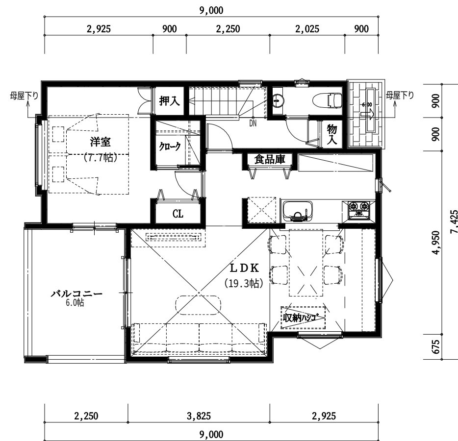
2階 平面図
